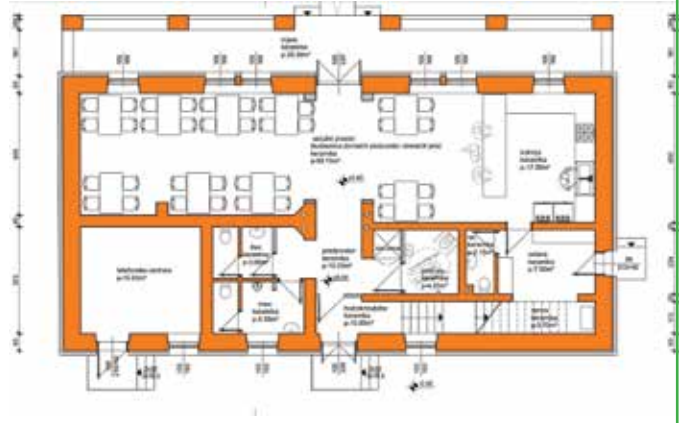
Projektno rješenje prostora
